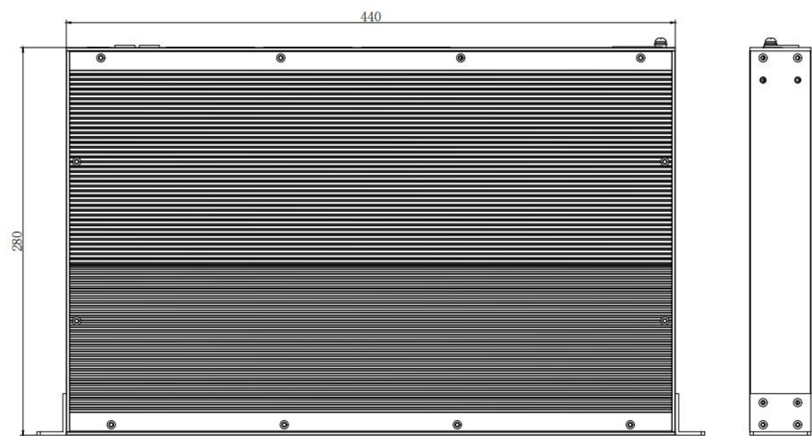
24 口机型
